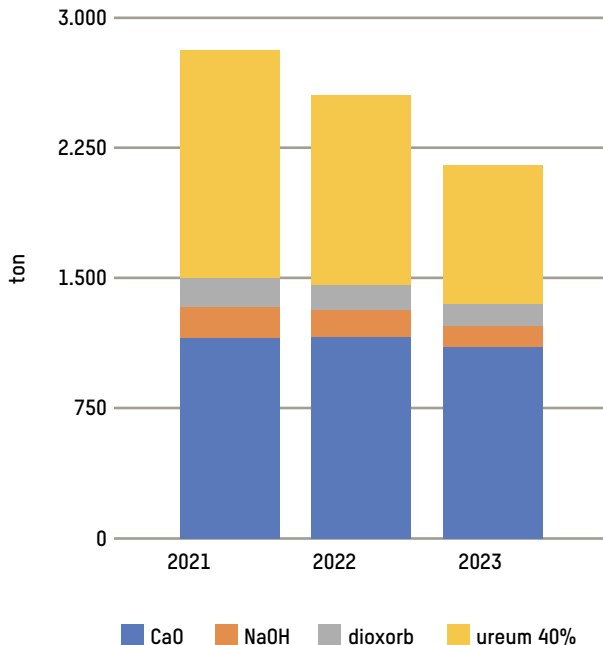
GRONDSTOFFEN AFVALENERGIECENTRALE
